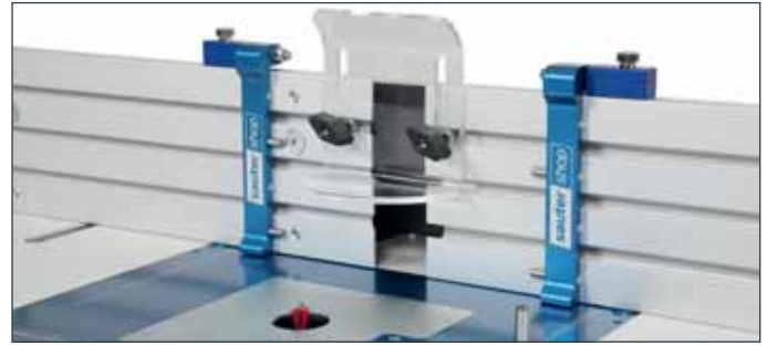
sauter Schwinganschläge
