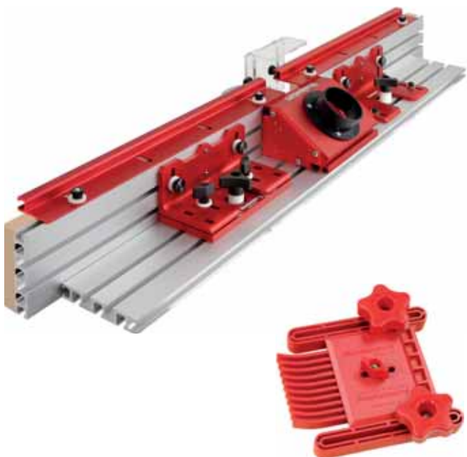
Druckkämme VPFB
