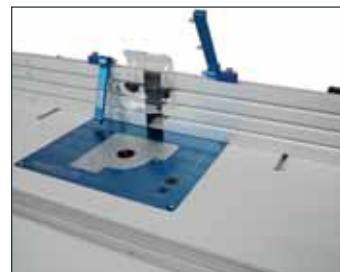
Schwinganschläge bei Nicht- gebrauch einfach wegklappen
